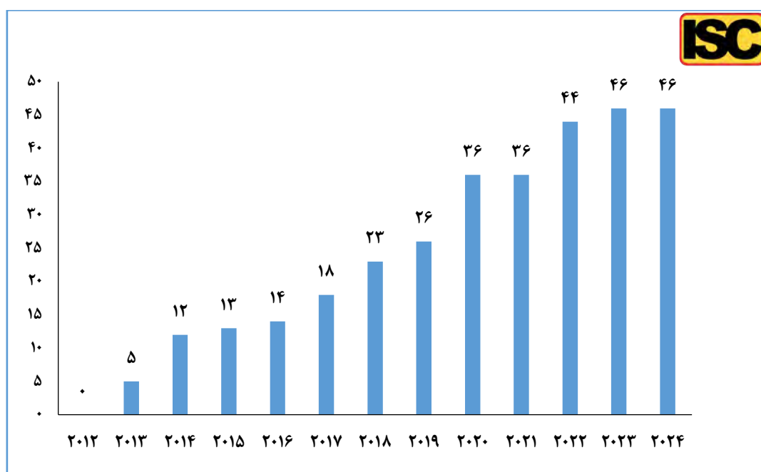
نمودار ۱. تعداد دانشگاه‌های ایران در نظام رتبه‌بندی لایدن تا سال ۲۰۲۴
